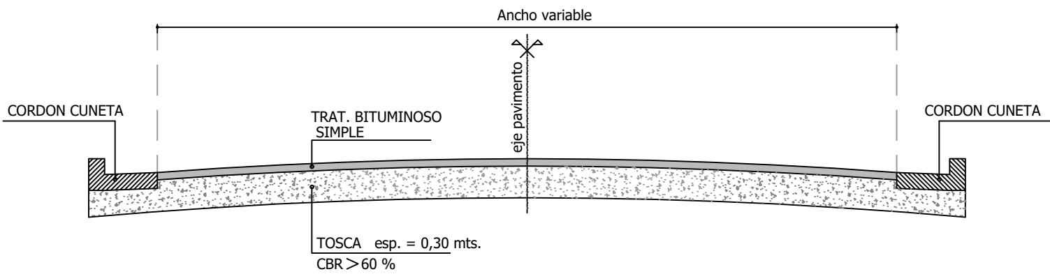
detalle PERFIL TIPO CALLE ESCALA 1 / 50
