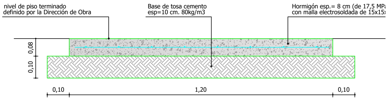
detalle de VEREDA ESCALA 1 / 10
