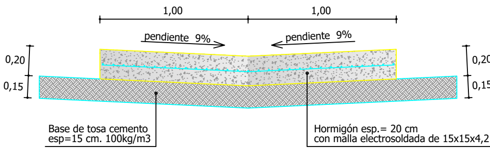
detalle BADEN de HORMIGÓN ESCALA 1 / 25
